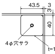
A部: 穴サラ付きプレート
