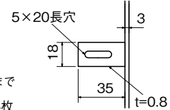
B部: 長穴付きプレート
