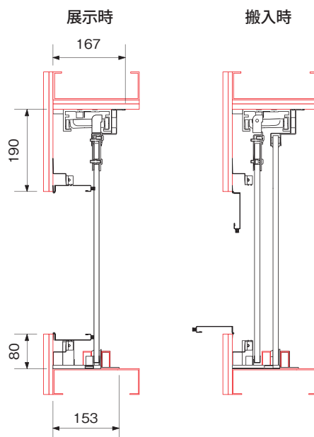
納まり図
