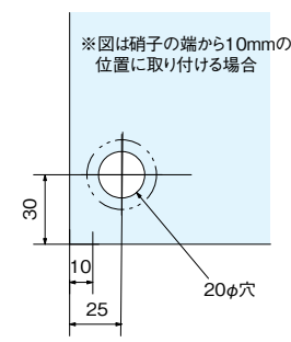
・硝子の加工図
