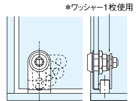
・八万ロック使用時の状態図
