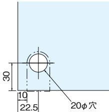
・硝子の加工図
