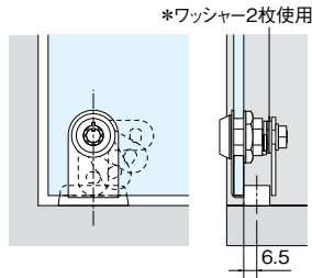
・八万ロック使用時の状態図
