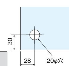
・硝子の加工図
