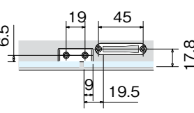
・YDロック使用時の状態図
