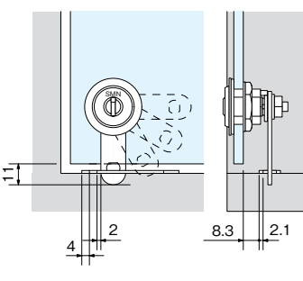
・YDロック使用時の状態図
