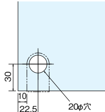
・硝子の加工図
