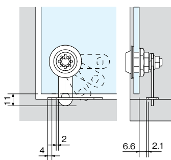
・八万ロック使用時の状態図
