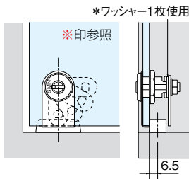
・硝子の加工図
