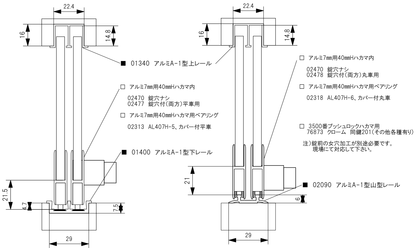
プラン図 No.01340-01400,02090
