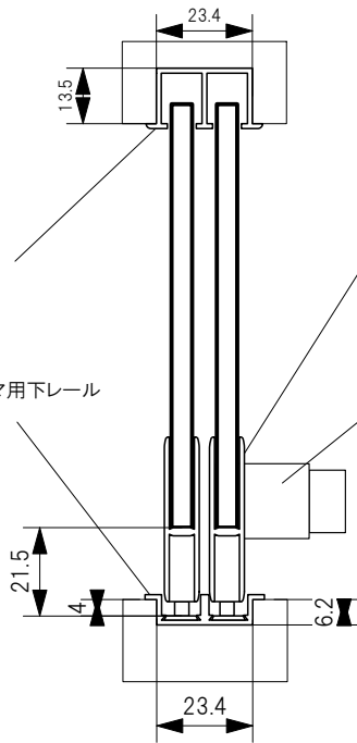
プラン図 No.02189-00990
