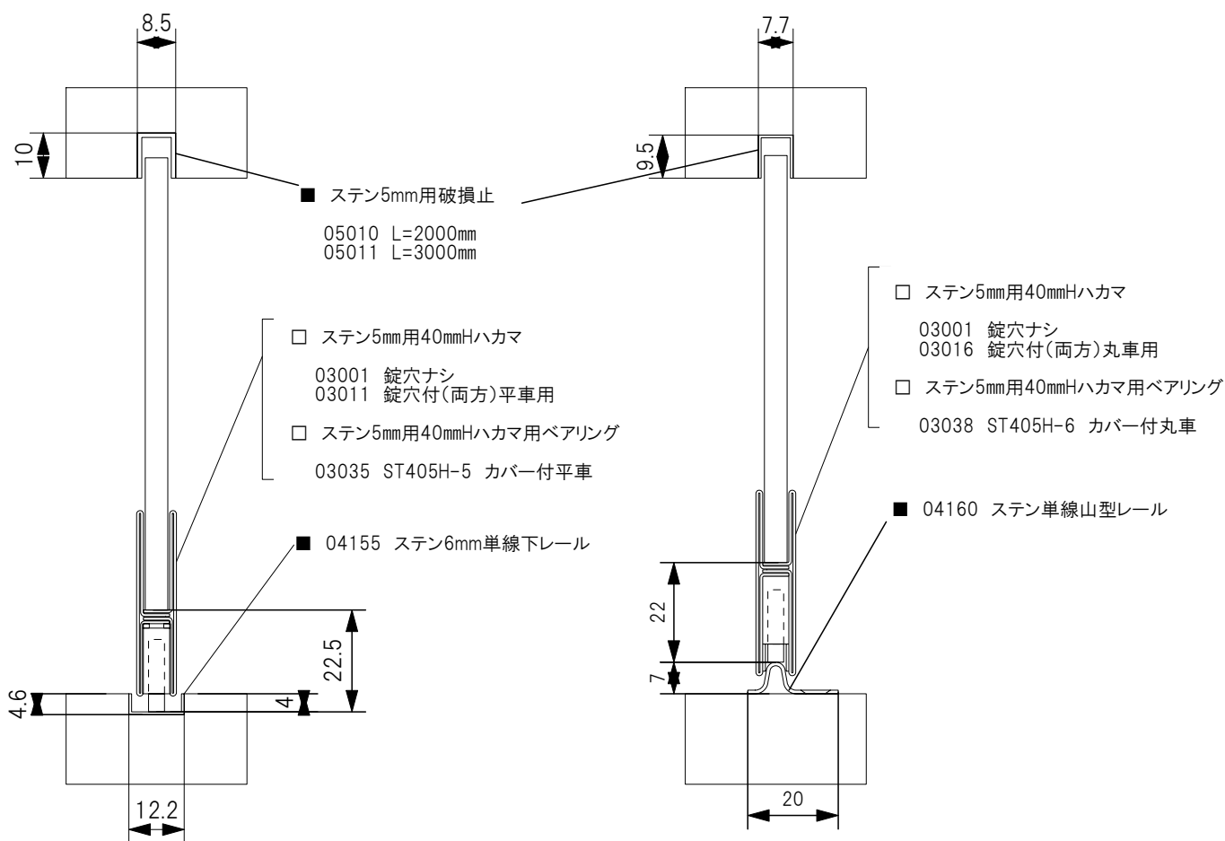
プラン図 No.05010-04155,04160
