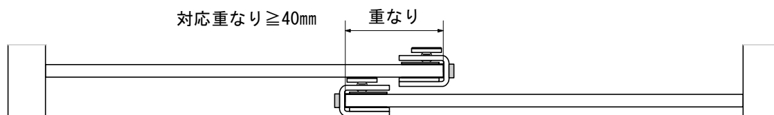
上面図
