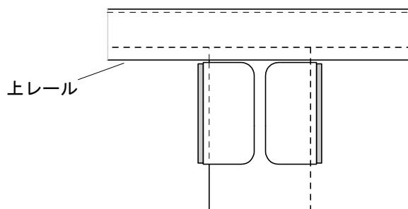
正面図
