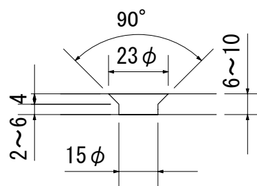
ガラス加工図
