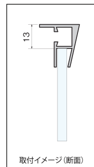
取付イメージ(断面)
