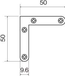
隅止金具
