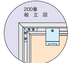
取付イメージ(断面)
