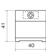
吊金具
