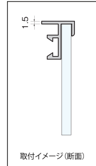
隅止金具
