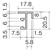
220番鏡枠
