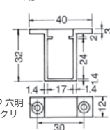
上用ソケット
