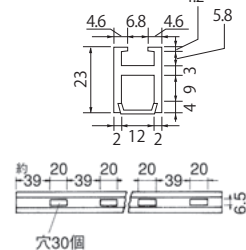
角柱 (正面側)
