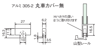
図 2 5mm用30mmHハカマ用取付車
