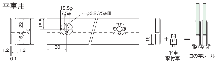
図1 5mm用40mmHハカマ
