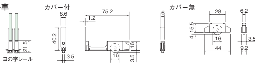
図2 5mm用40mmHハカマ用取付車
