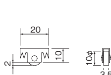
図 4 5mm用25mmHハカマ用取付車
