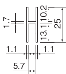
図 3 5mm用25mmHハカマ
