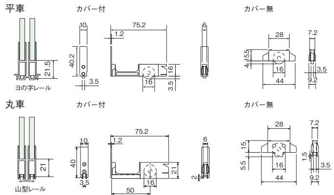
図2 7mm用40mmHハカマ用取付車
