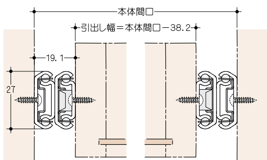
取付図
