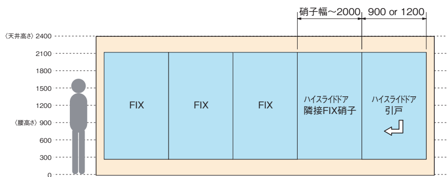
〈外形図・横断面図〉
