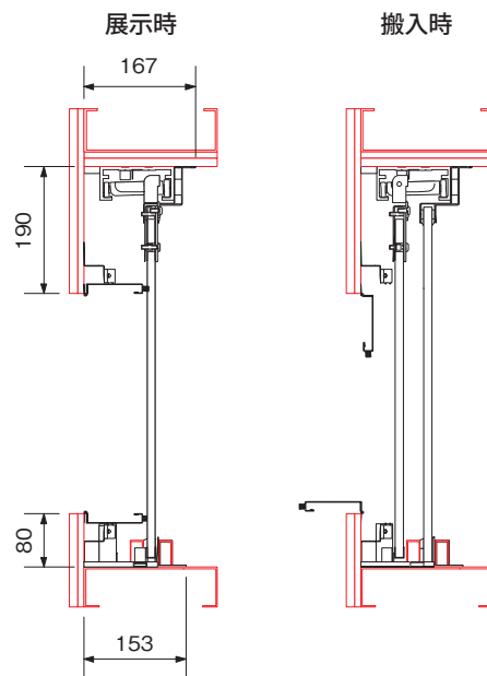
納まり図
