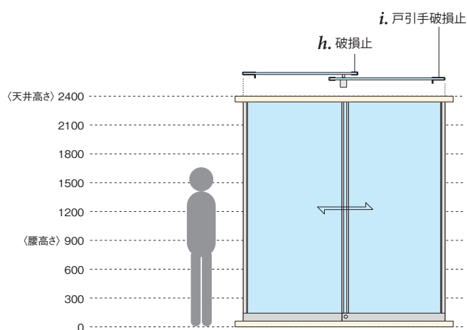
〈外形図・横断面図〉
