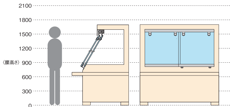
〈外形図〉
