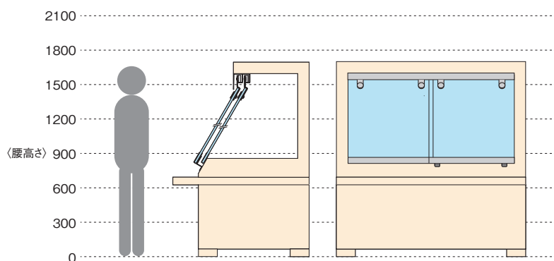
〈外形図〉
