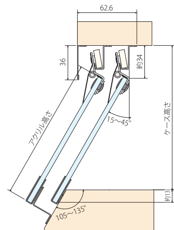
〈横断面図〉
