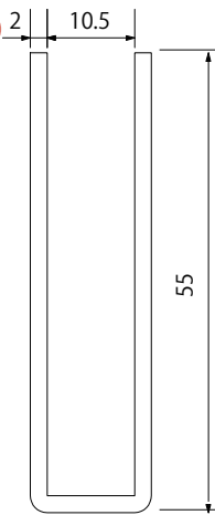
厚口破損止 10 x 55
