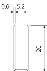
5-2 深型破損止 20mm
