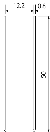
12mm用50mm 深型破損止
