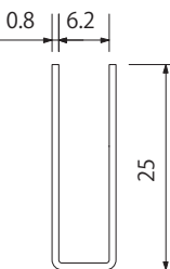
5mm 用 25mm 破損止
