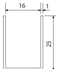
パーティションチャンネル 2518
