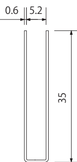
5-2 深型破損止 35mm
