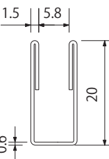
5mm フレーム破損止
