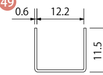
12mm チャンネル HL
