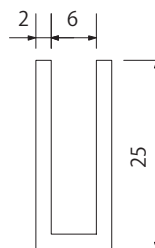
厚口破損止 5 x 25
