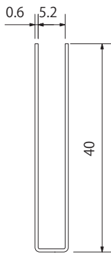
5-2 深型破損止 40mm
