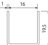
40 号 12mm 単線上レール
