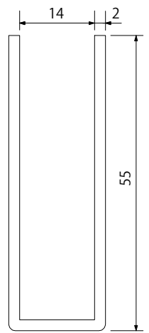
厚口破損止 12 x 55
