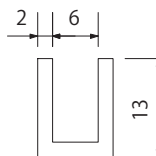
厚口破損止 5 x 13
