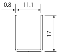
6mm マルチ上レール S
