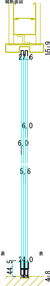
縦断面図
