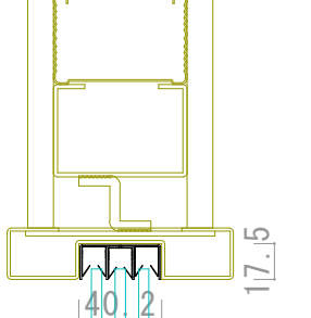
縦断面図
