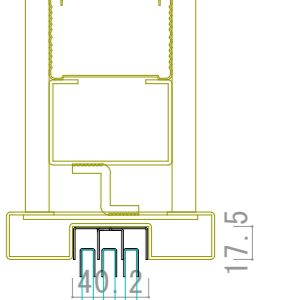
縦断面図
