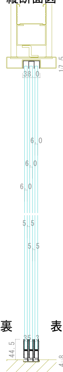
縦断面図
