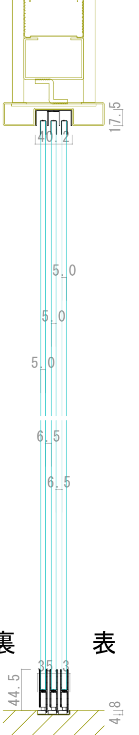
縦断面図
