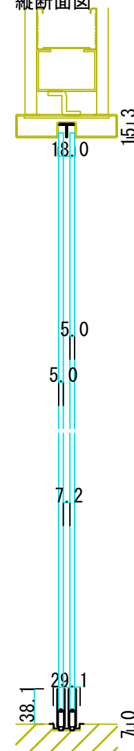
縦断面図
