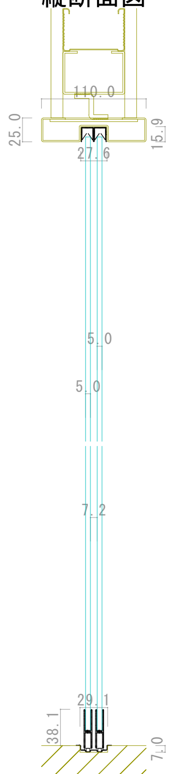
縦断面図
