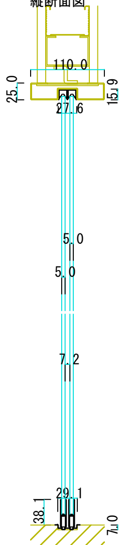
縦断面図
