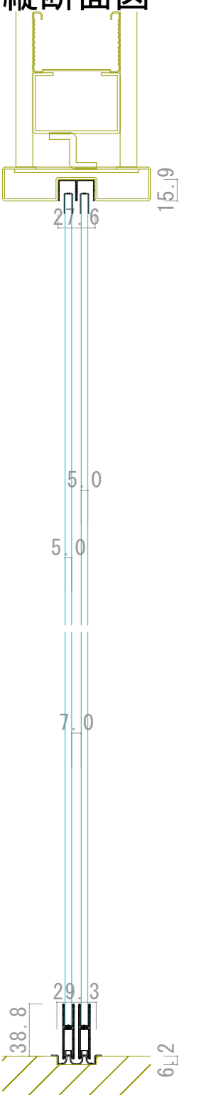
縦断面図
