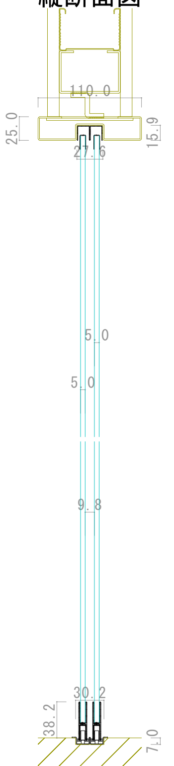
縦断面図
