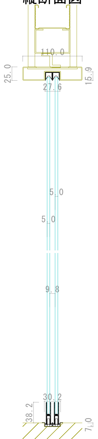
縦断面図
