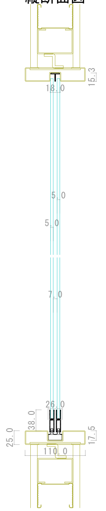
縦断面図
