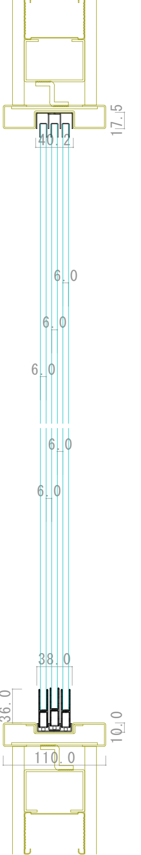
縦断面図
