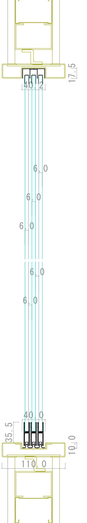
縦断面図
