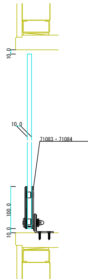
B-B断面図
