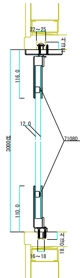
A-A断面図
