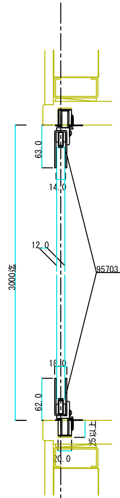
A-A断面図
