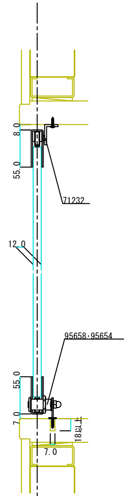
B-B断面図
