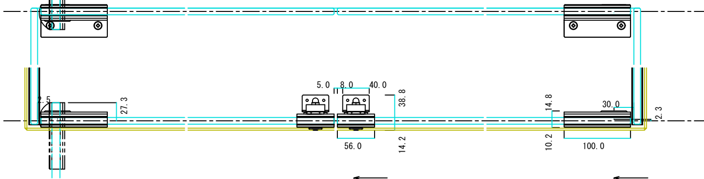
C-C断面図
