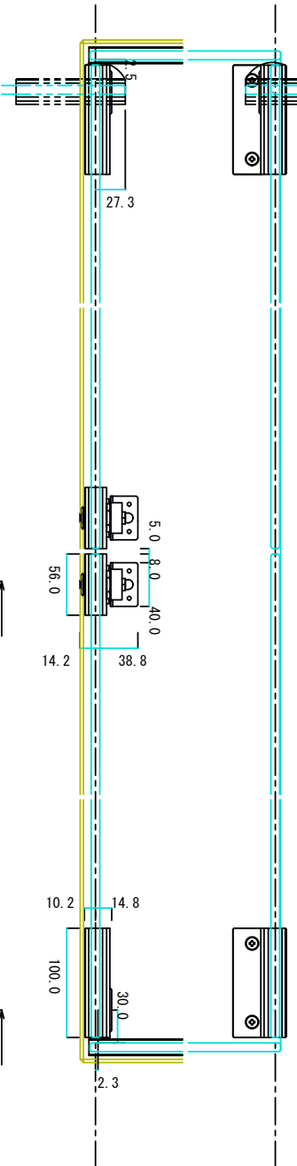
C-C断面図
