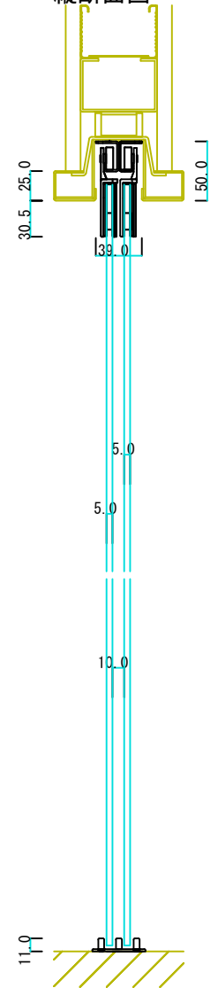
縦断面图
