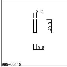
正面図
