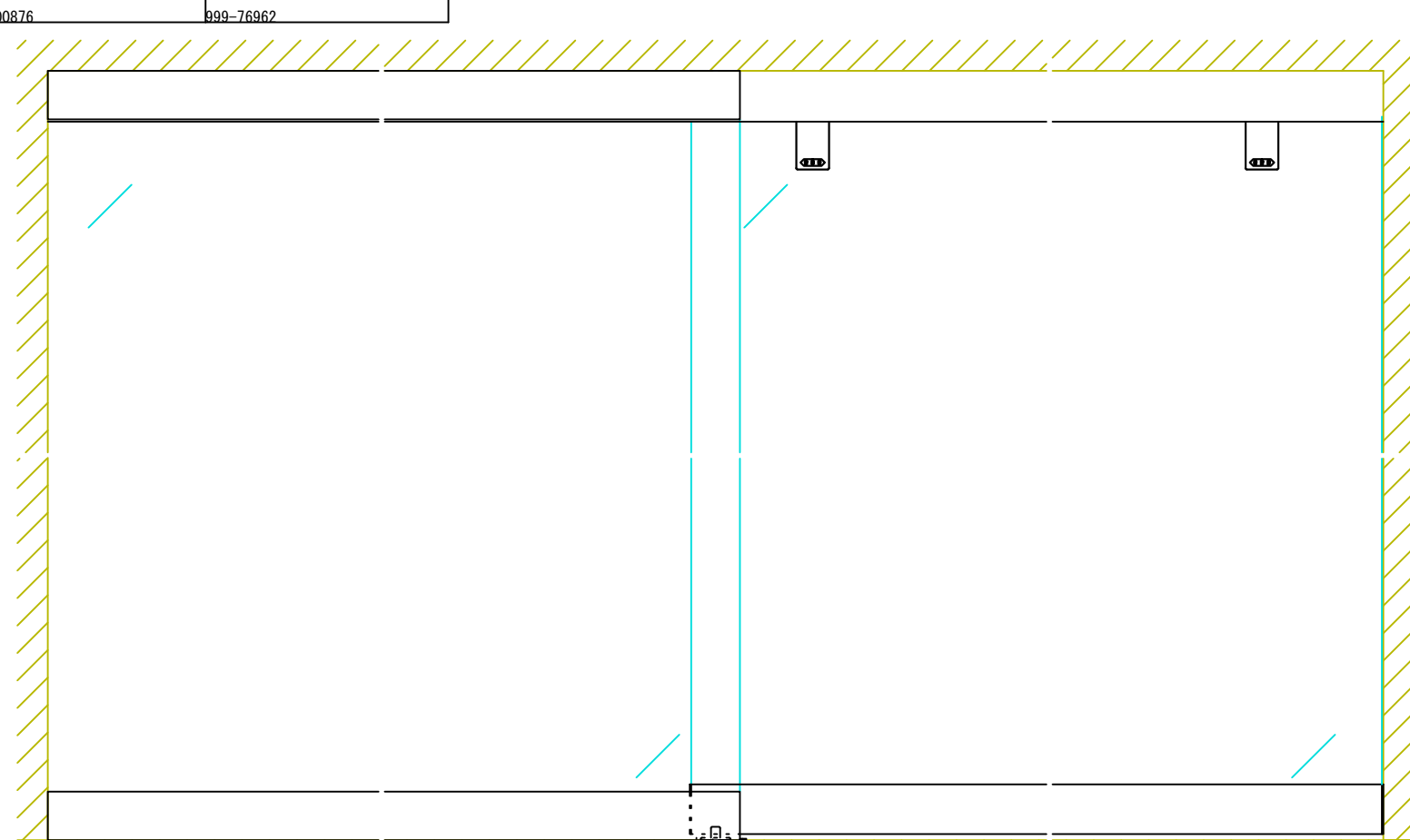
正面図
