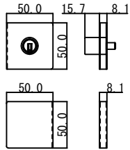
正面図
