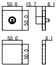
正面図
