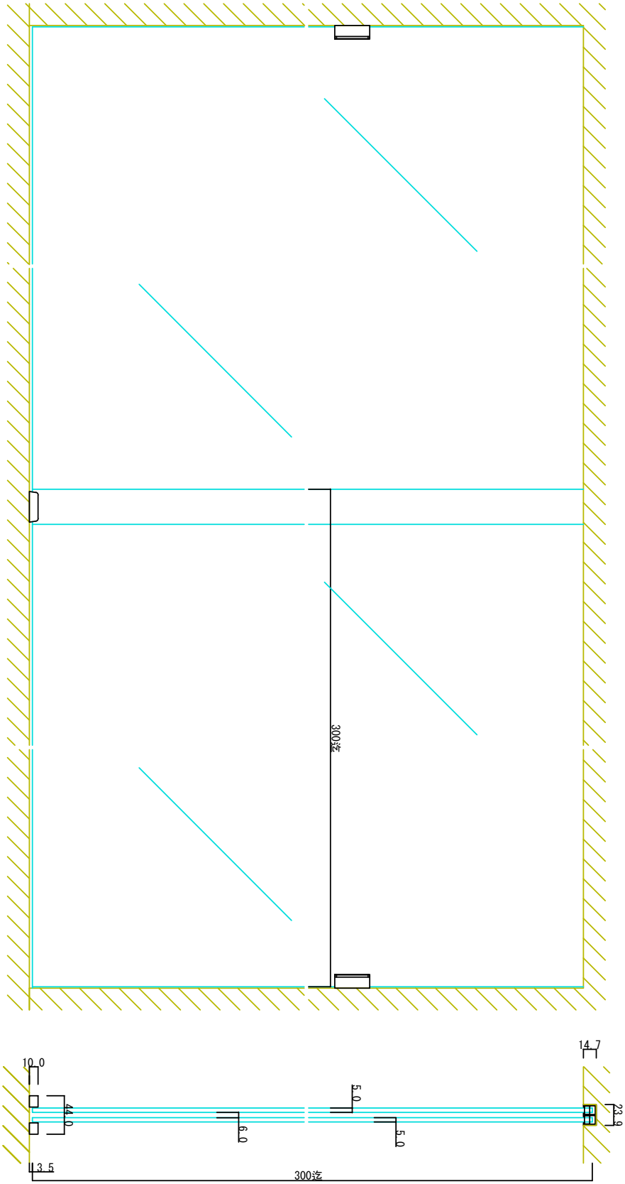
正面図
