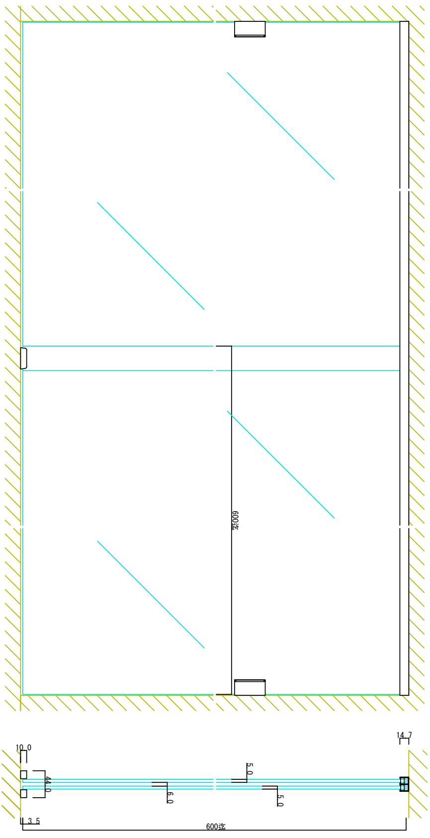
正面図
