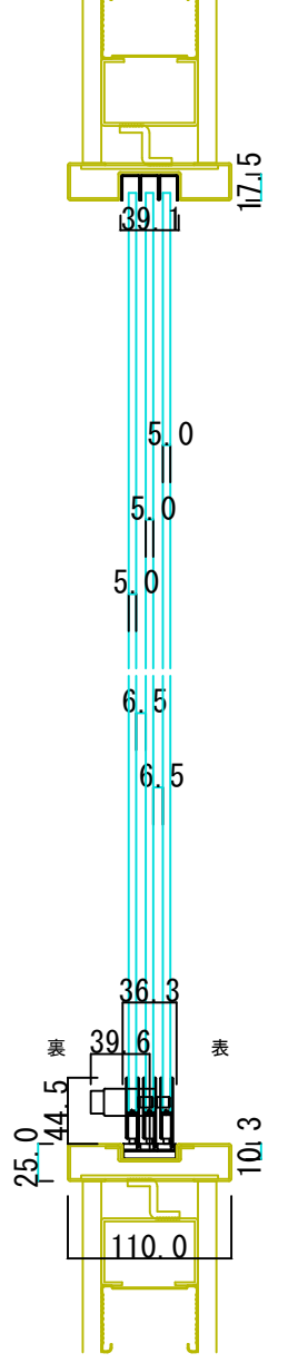
縦断面図
