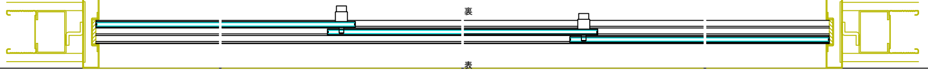
横断面図
