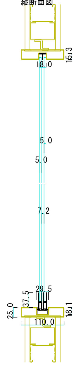
縦断面図
