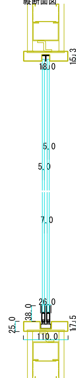
縦断面図
