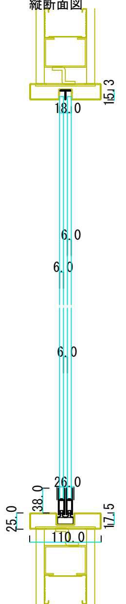
縦断面図
