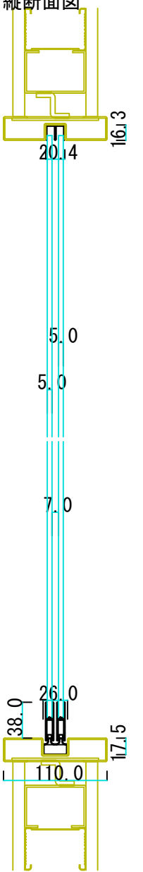
縦断面図
