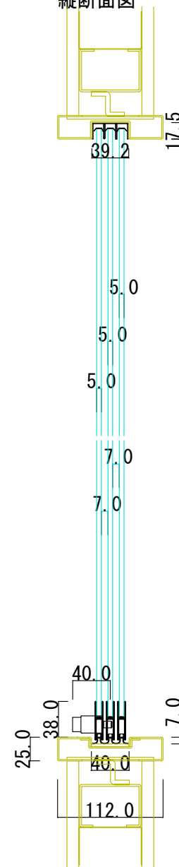
縦断面図
