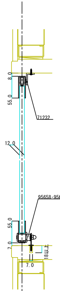
B-B断面図
