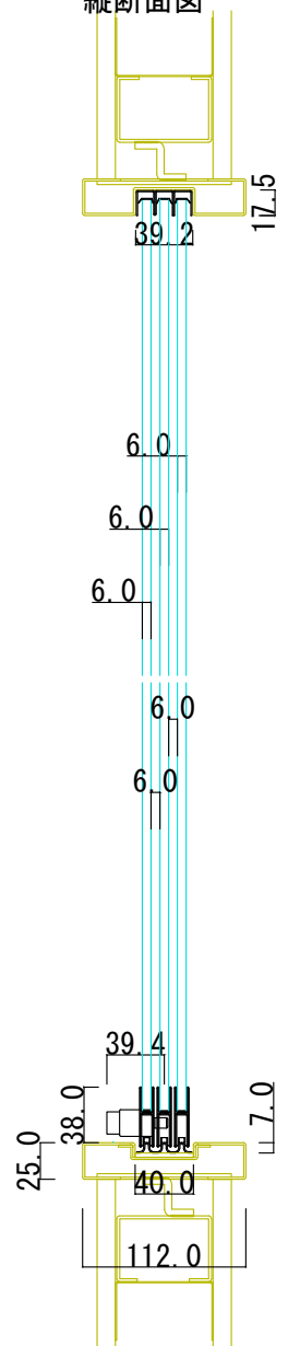
縦断面図
