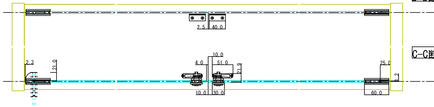
D-D断面図
